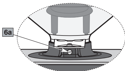
Detail A (Kaffeebohnenbehälter)
